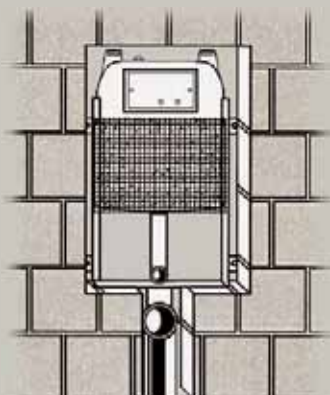
INCASSO A MURARE
