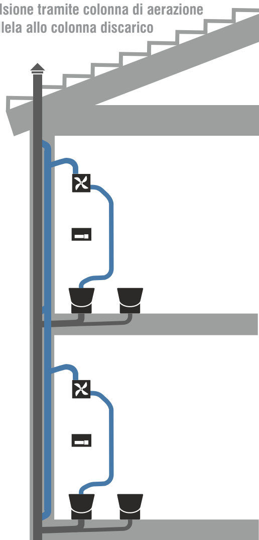
Esempio di impianto di scarico con ventilazione tramite colonna parallela alla colonna di scarico
