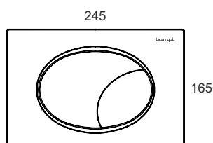
Spessore 12 mm.
