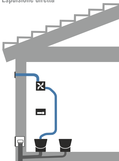
Esempio di impianto di scarico con ventilazione tramite valvola di aerazione
