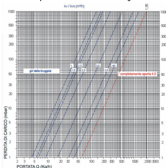
Curva perdite di carico detentori di regolazione
